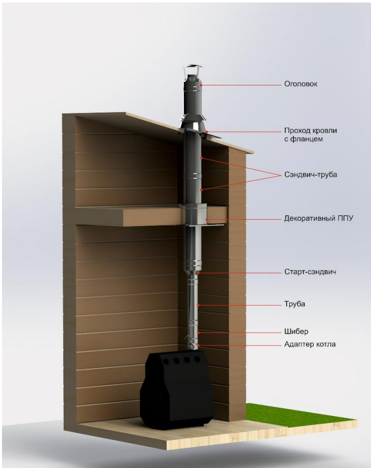
Рис.6 Двустенный вертикальный дымоход с проходом через потолочное перекрытие и кровлю, при вертикальном выходном патрубке котла.
