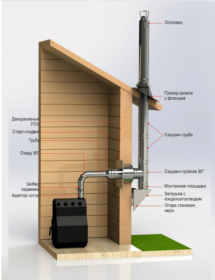
Рис.9 Двустенный вертикальный дымоход на внешней стороне стены с проходом через стену и кровлю при вертикальном выходном патрубке котла.
