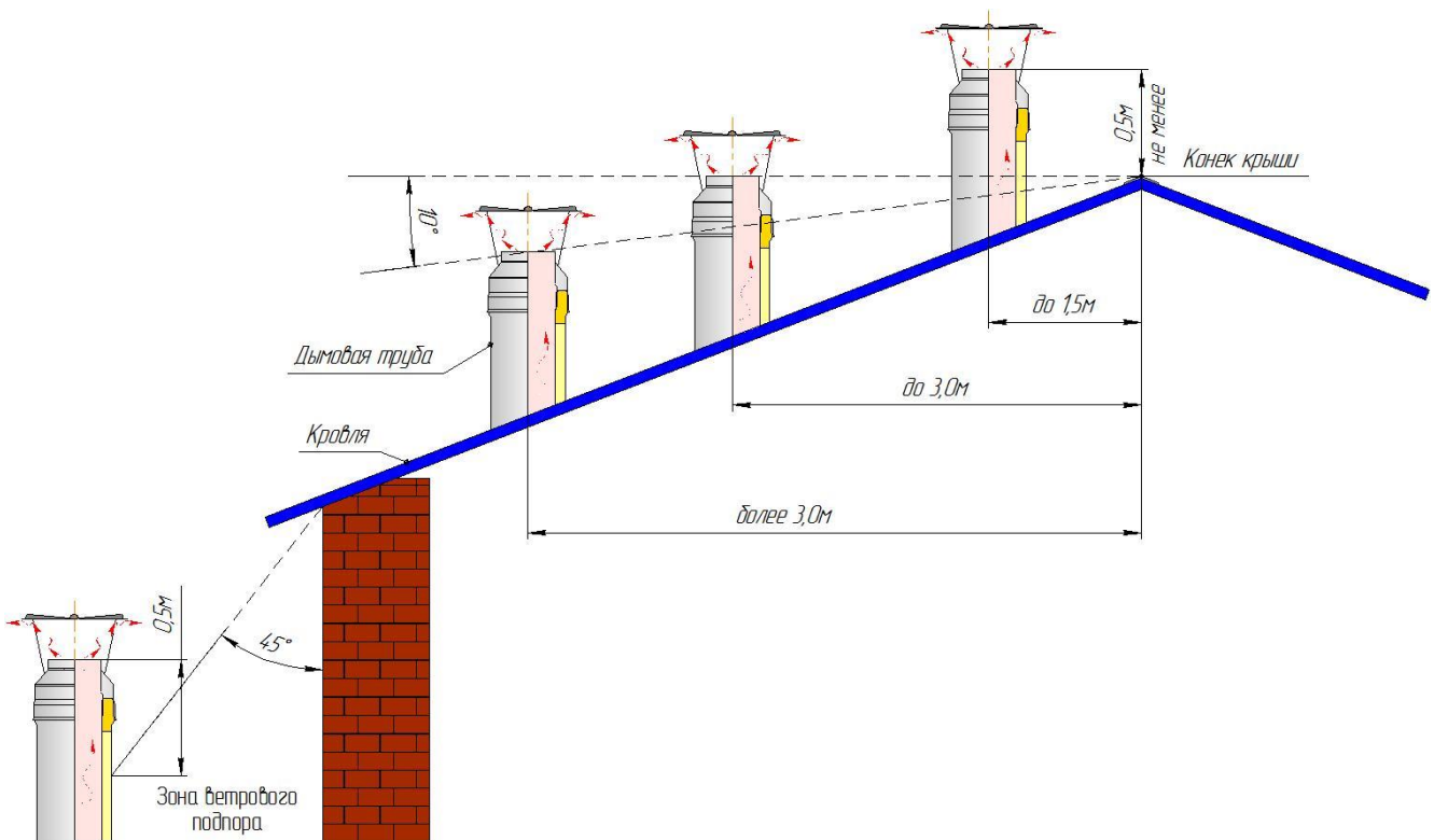
Рис. 4. Схема определения высоты наружной части дымовой трубы. (Согласно СНиП 41-01-2003.)
