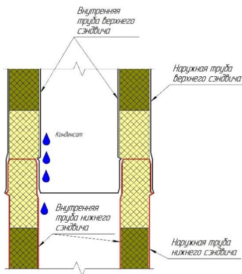
Рис. 5. Схема сборки двухконтурной трубы («сэндвич»). (Разрез по вертикальной оси «сэндвича».)
