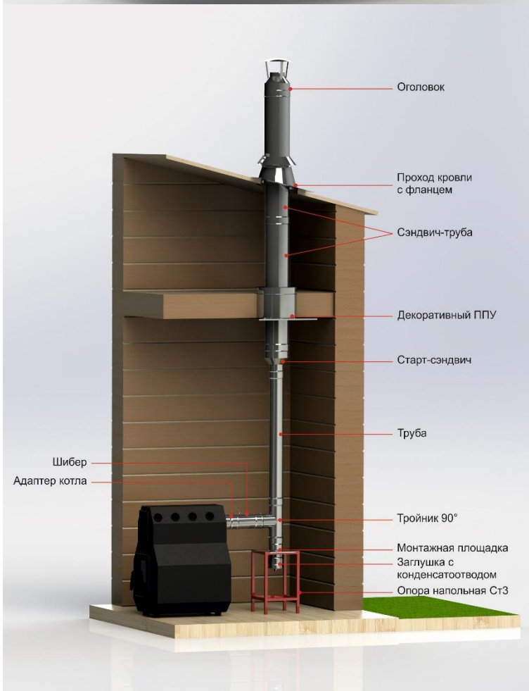
Рис.7 Двустенный вертикальный дымоход с проходом через потолочное перекрытие и кровлю, при горизонтальном выходном патрубке котла.
